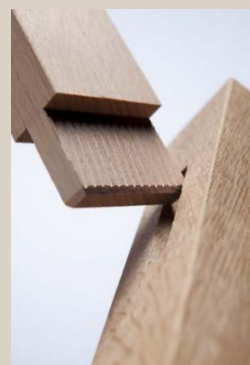
接合部（ホゾ）に施された独自の創意工夫が強度の要。
